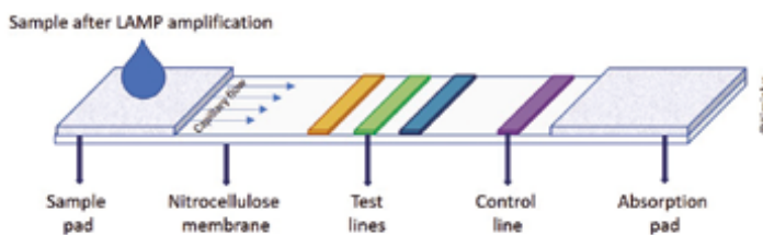
Vue schématique simplifiée du test bandelette O2DIAG, permettant un diagnostic rapide et fiable de l'agent infectieux ciblé
